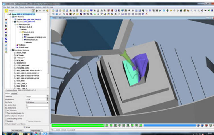
CAM プログラマーの Jake Oliveira が、ペリカットの NC シミュレーションを、DMG の 5 軸マシニングセンターに適用している
